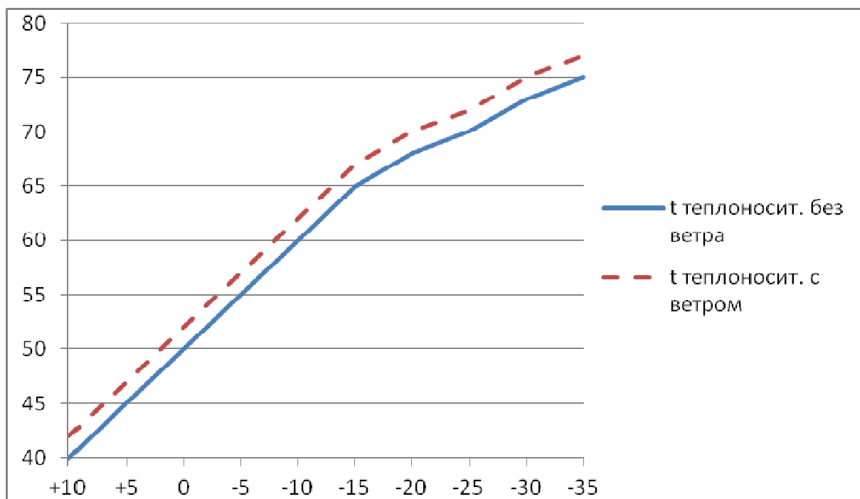
Рисунок 2. График зависимости температуры теплоносителя в подающем трубопроводе на выходе из котельной от температуры наружного воздуха
